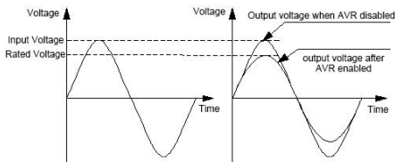
Fig. FC-2 AVR Function
