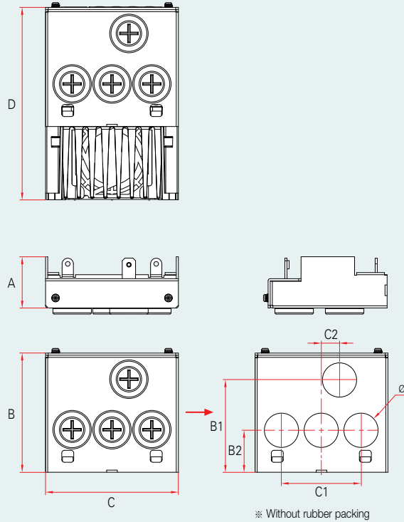
Drive + Conduit
