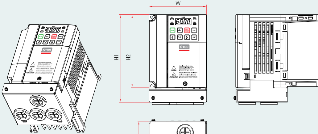
Drive + Conduit
