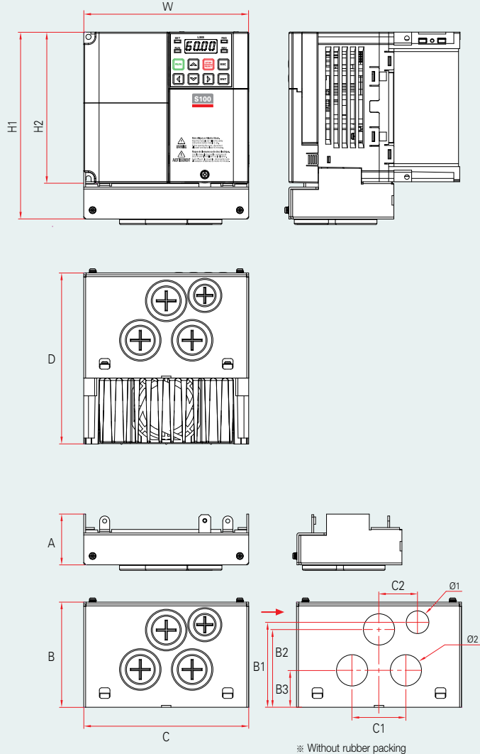
Drive + Conduit
