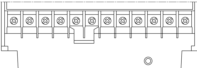
ATV31HD11M3X, HD15M3X, HD11N4, HD15N4, HD11S6X, HD15S6X
